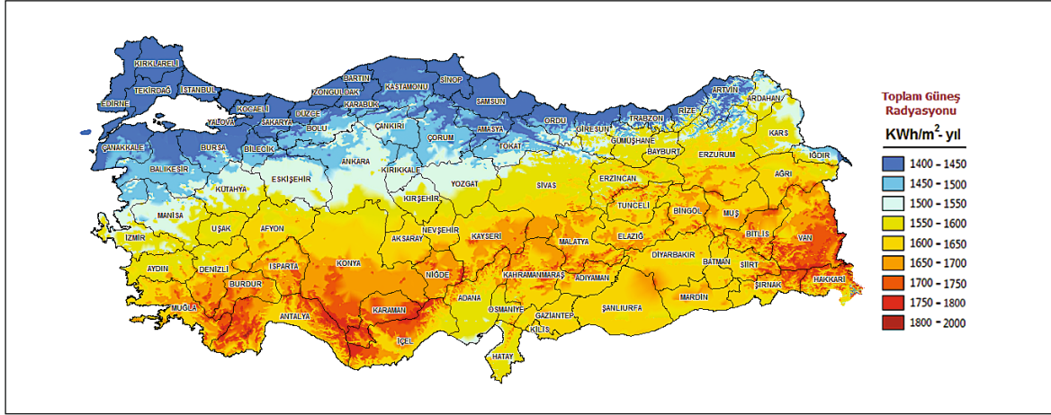
Şekil 219: Türkiye güneş enerjisi potansiyeli
