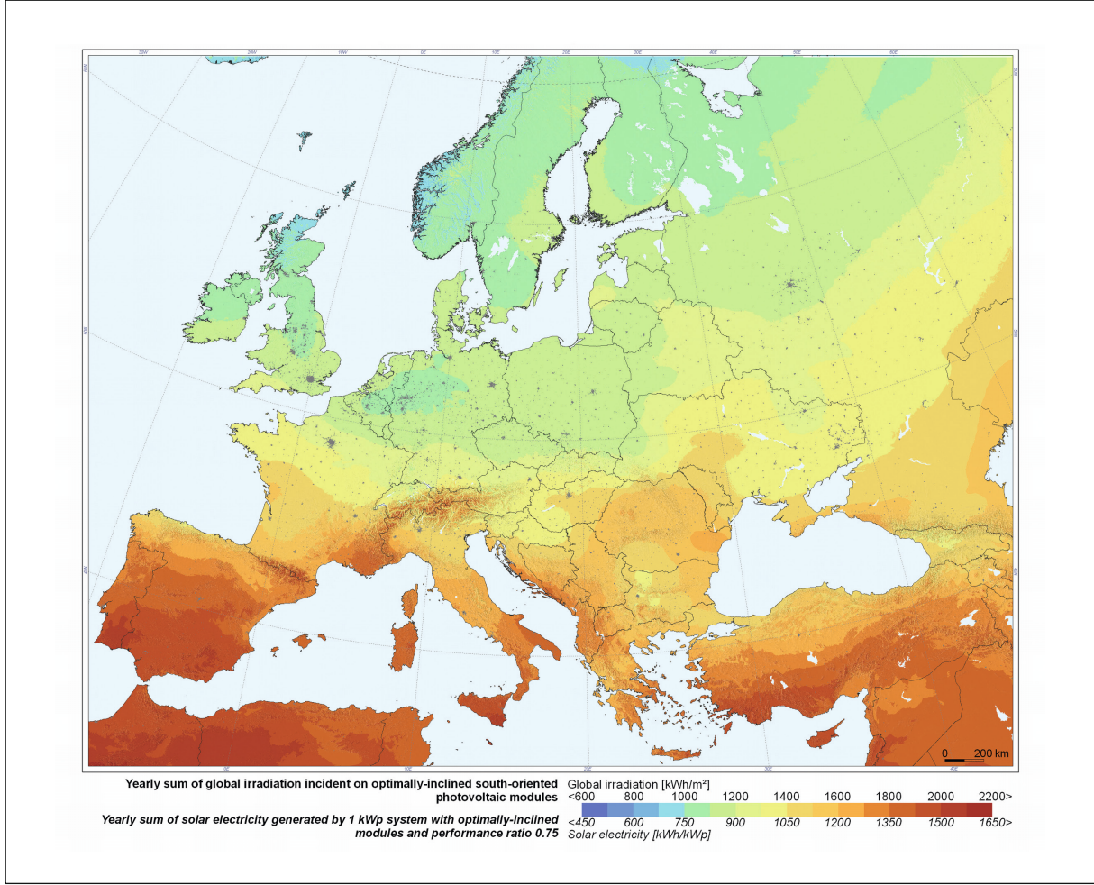
Şekil 218: Avrupa ülkelerinde güneş enerjisi potansiyeli
