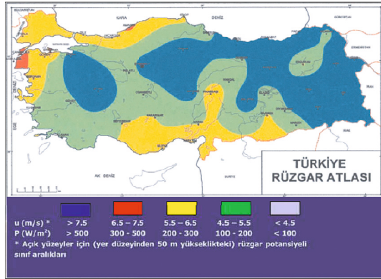
Şekil 214:Türkiye rüzgâr enerjisi potansiyeli
