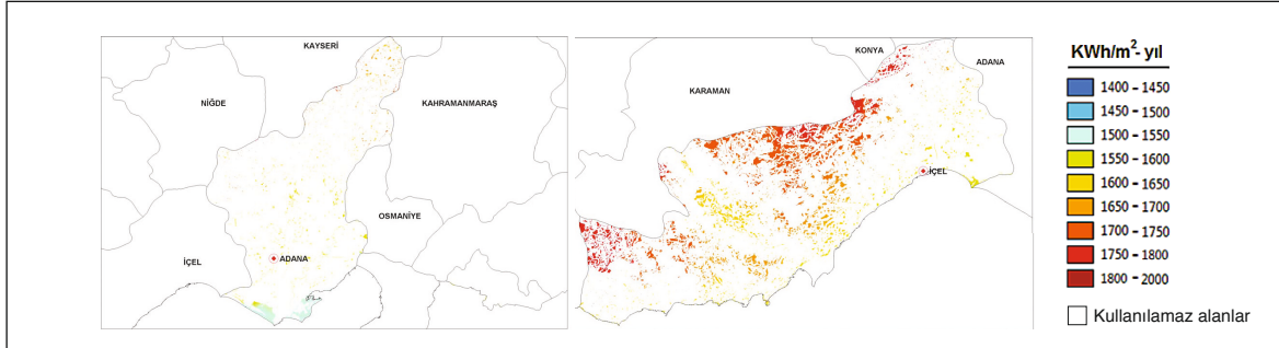
Şekil 220: Güneş termik santrali kurulabilir alanlar
