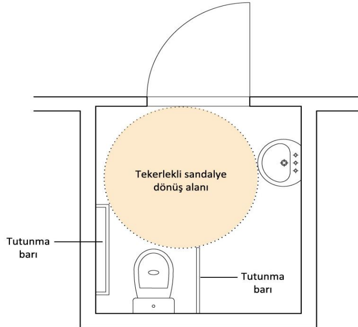
Resim 24: Engelli Tuvaleti Plan Şeması
