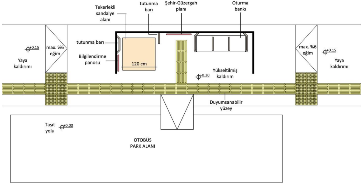
Resim 53: Otobüs Durağı Plan Şeması
