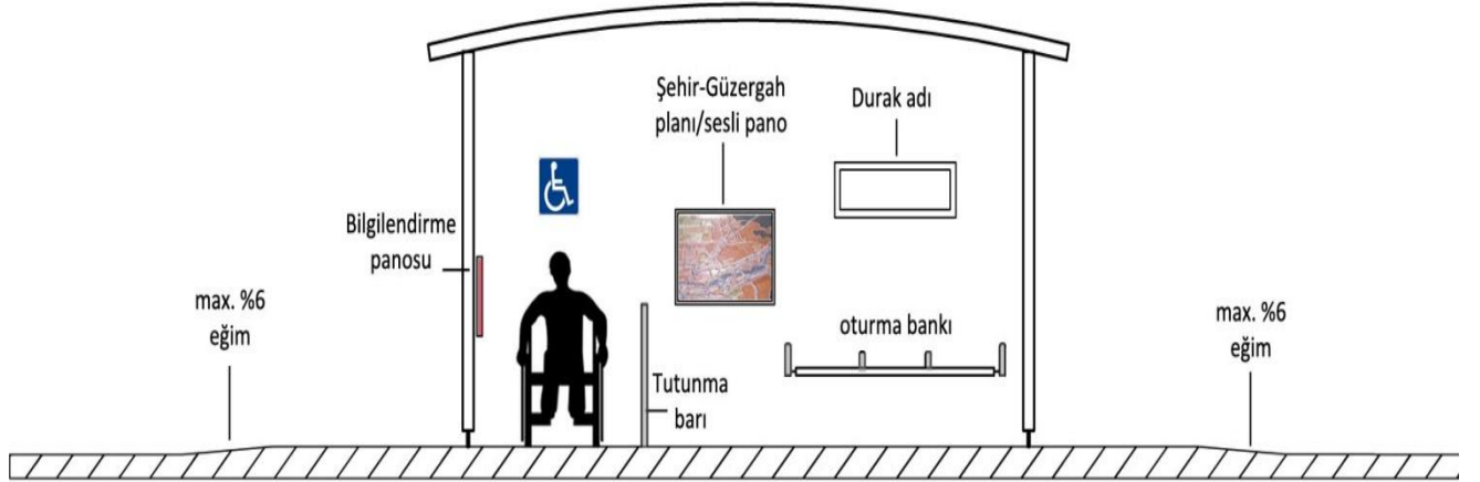
Resim 56: Otobüs Durağı Görünüş Şeması
