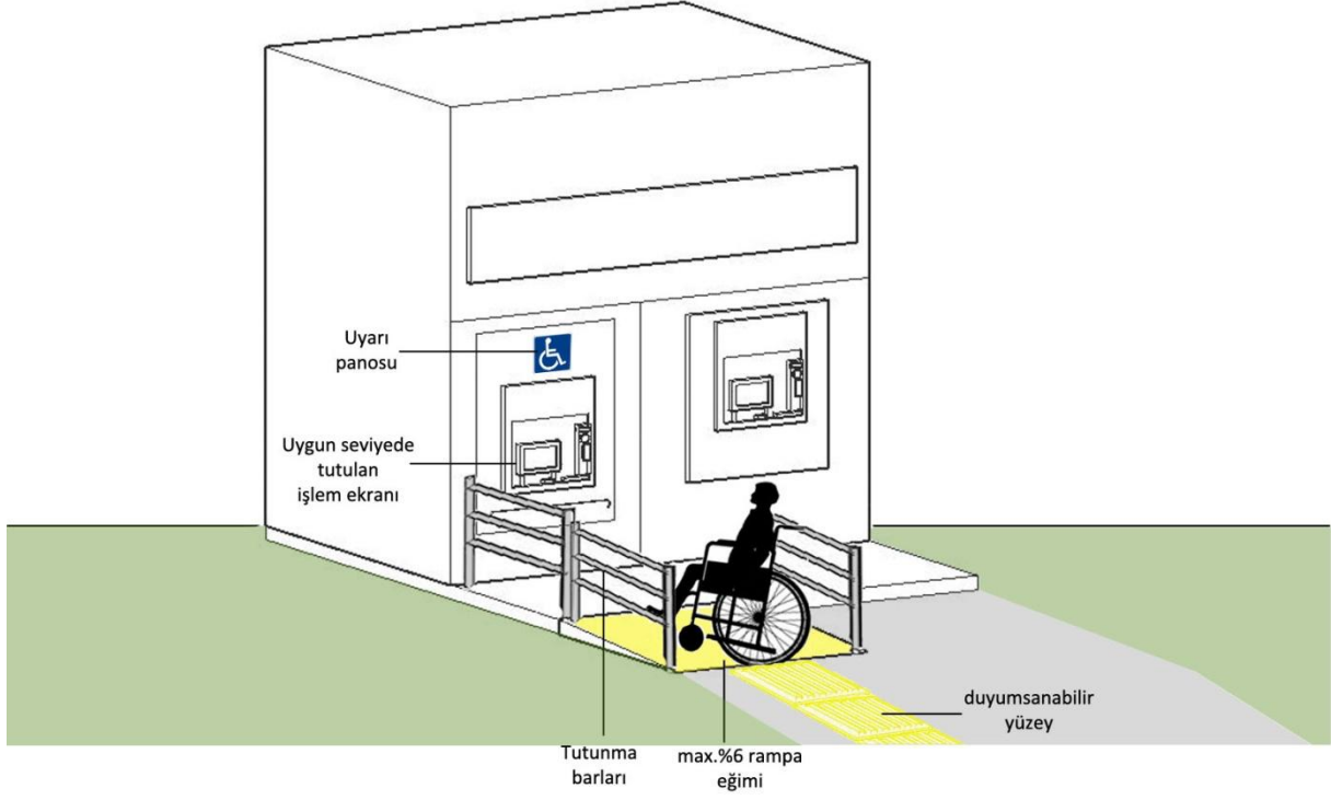
Resim 61: Engelli PTT Birimi Perspektif
