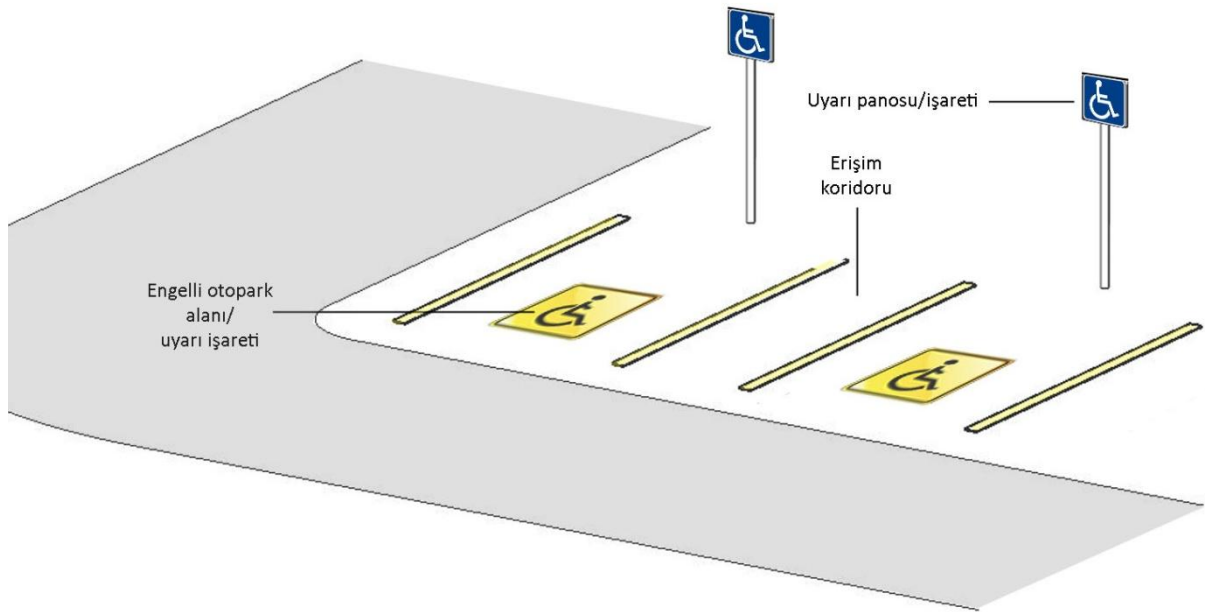
Resim 34: Engelli Otopark Şeması
