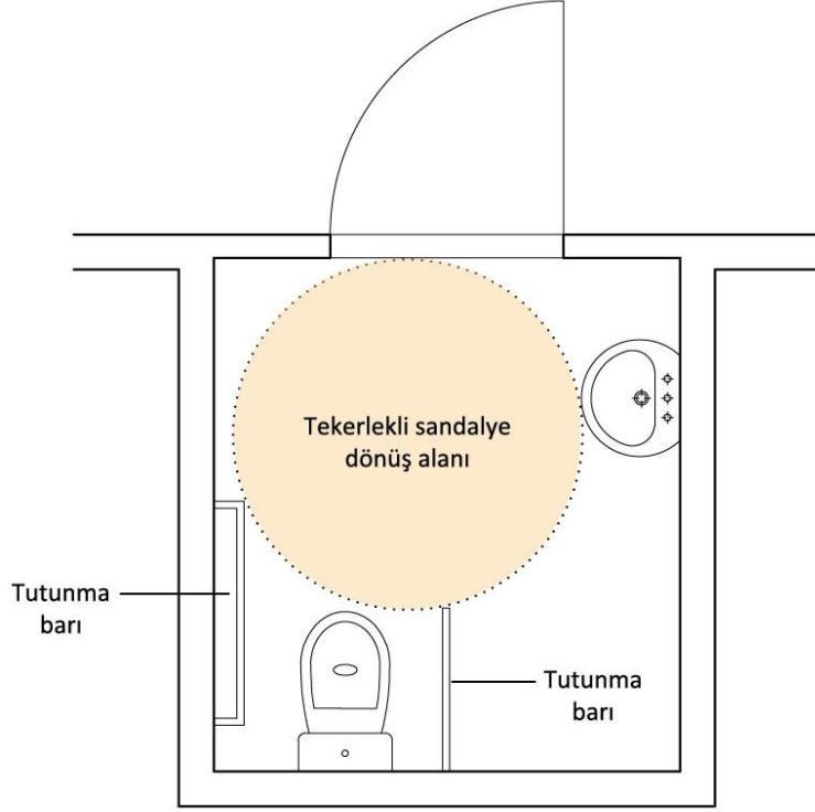
Resim 41: Engelli Tuvaleti Plan Şeması
