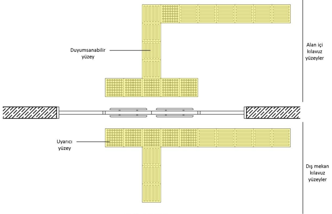
Resim 59: Duyumsanabilir Yüzeyler Plan Şeması
