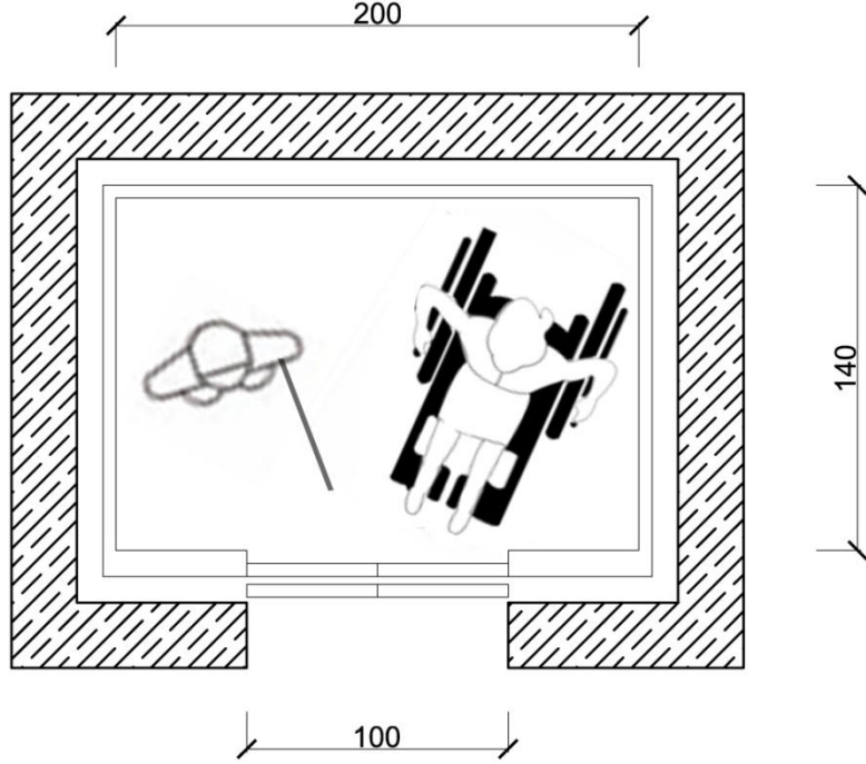
Resim 39: Engelli Asansörü Plan Şeması
