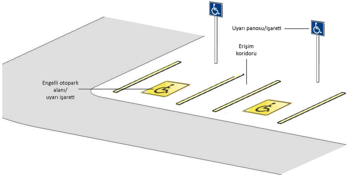
Resim 42: Engelli Otopark Şeması
