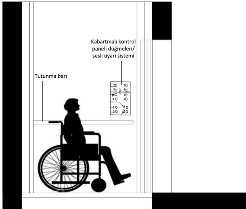
Resim 36: Engelli Asansörü Kesit Şeması
