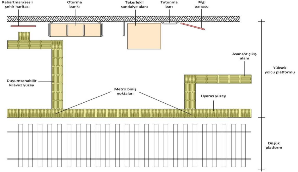
Resim 43: Metro İstasyonu Plan Şeması
