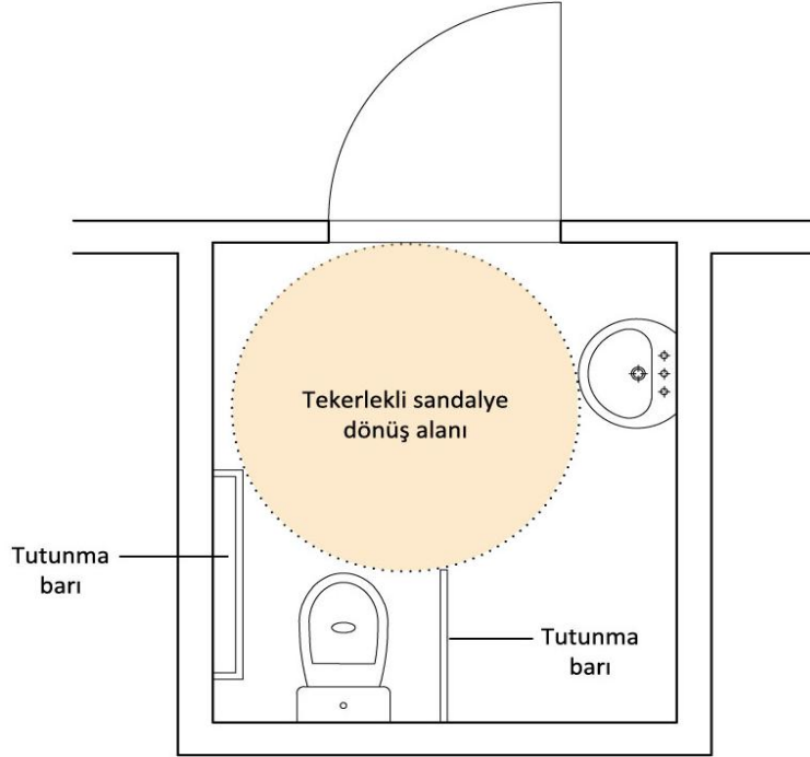
Resim 33: Engelli Tuvaleti Plan Şeması
