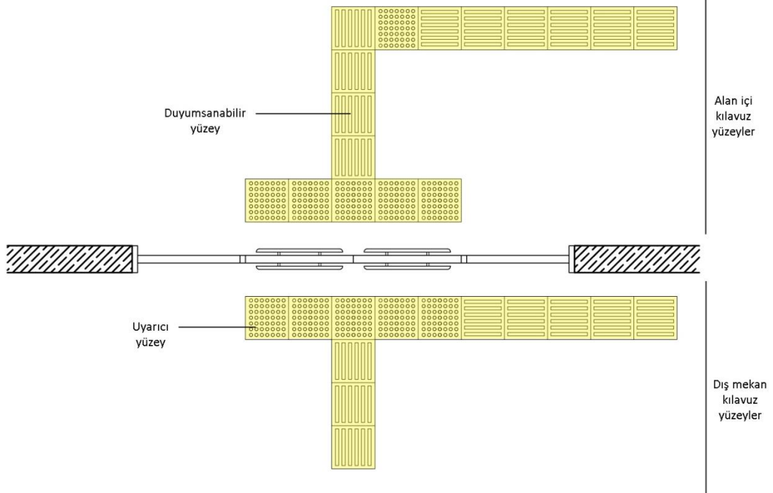
Resim 48: Giriş Kapısı Plan Şeması
