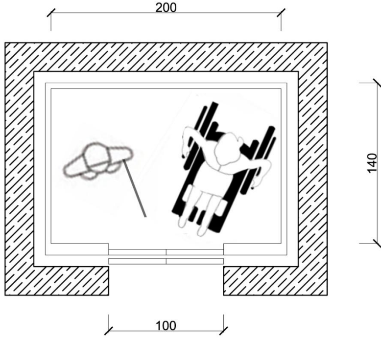
Resim 15: Engelli Asansörü Plan Şeması
