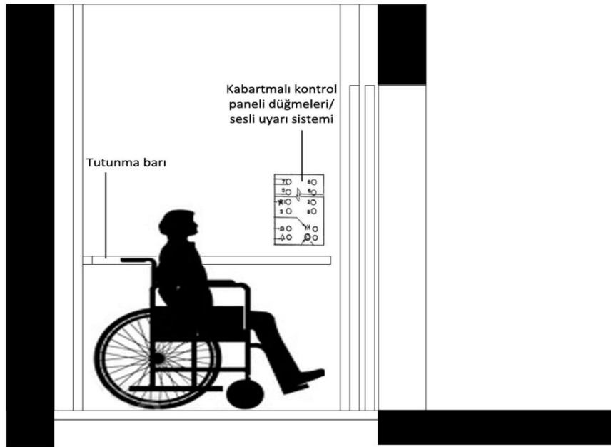
Resim 16: Engelli Asansörü Kesit Şeması
