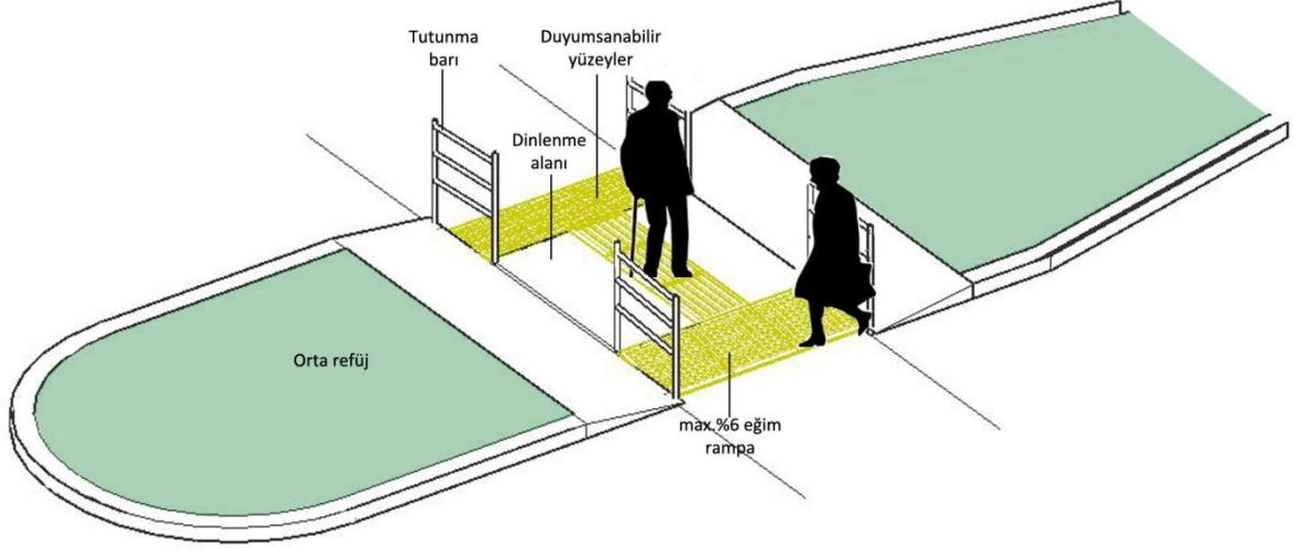
Resim 65: Geniş Refüjde Yaya Geçidi Perspektif
