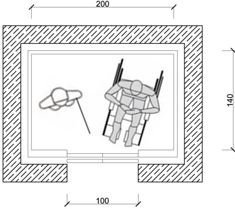
Resim 45: Engelli Asansörü Plan Şeması
