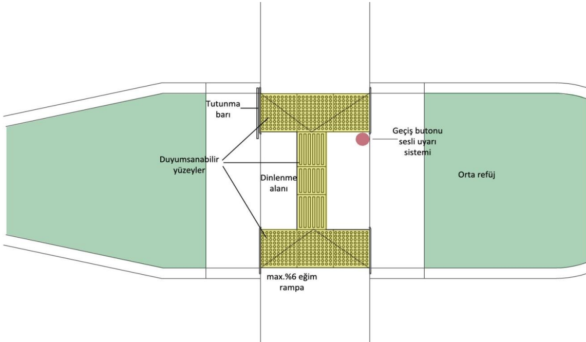
Resim 64: Geniş Refüjde Yaya Geçidi Plan Şeması
