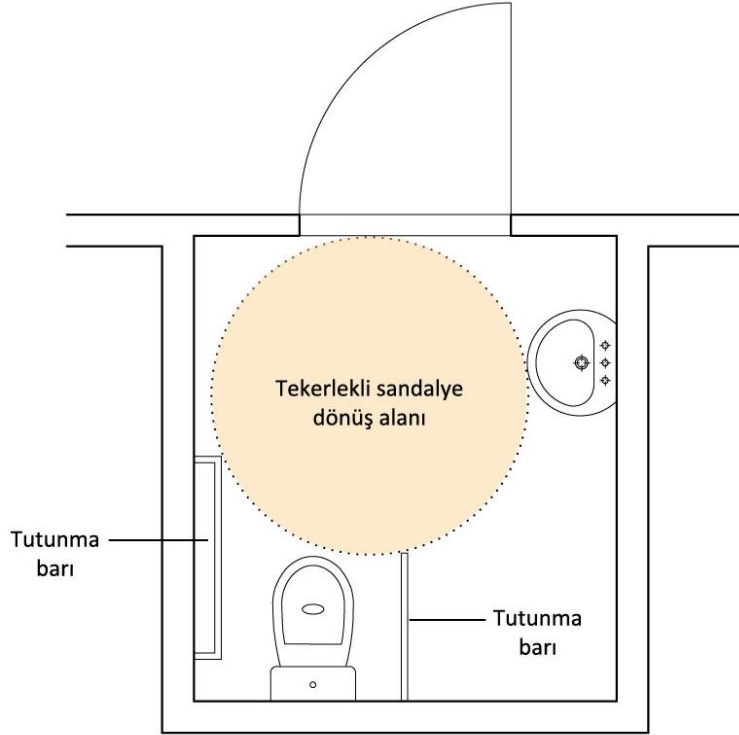
Resim 13: Engelli Tuvaleti Plan Şeması
