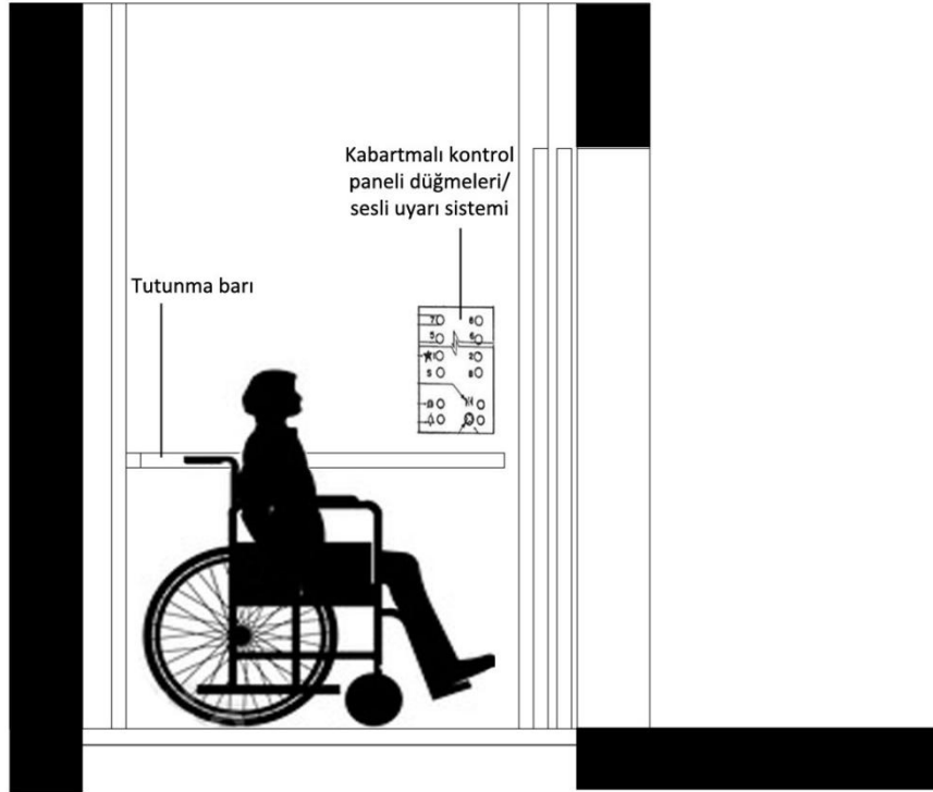
Resim 40: Engelli Asansörü Kesit Şeması
