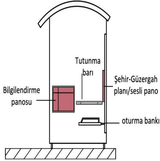
Resim 55: Otobüs Durağı Kesit Şeması
