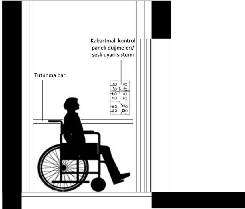
Resim 46: Engelli Asansörü Kesit Şeması
